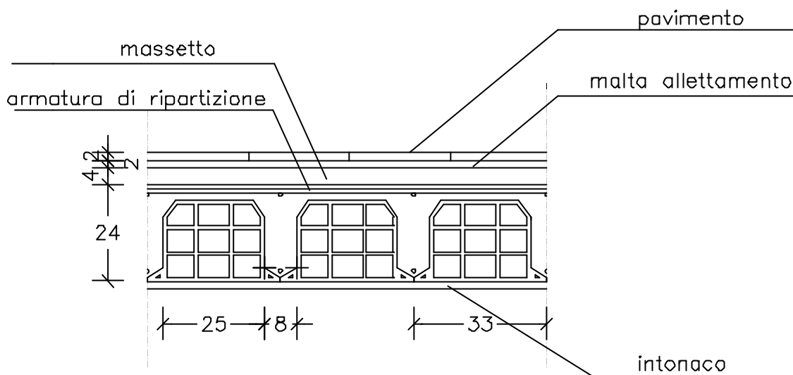
Fig.2.1 – Schema del solaio
